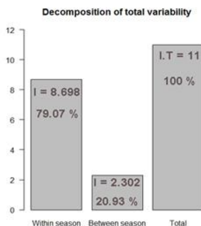
Figure 2: Décomposition de total variability
